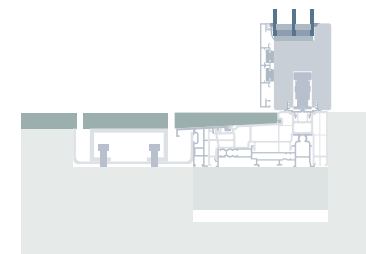
Dvižno drsna stena - poravnani prag (podnice)
