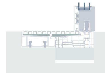
Dvižno drsna stena - poravnani prag (rešetka)
