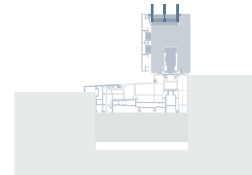
Dvižno drsna stena - klasični prag
