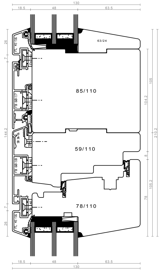
sestav po vertikali - FIX/DK
