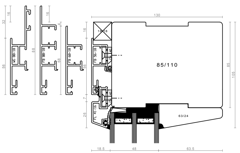
pokončnik in zgornji prečnik - fiksno okno
