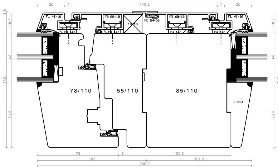
sestav po horizontali - DK/FIX
