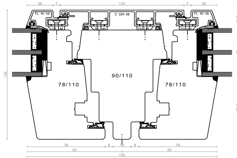
dvokrilno s pokončnikom - DK/DK
