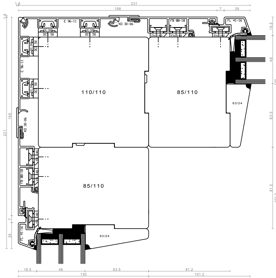
vognalni sestav - FIX/FIX
