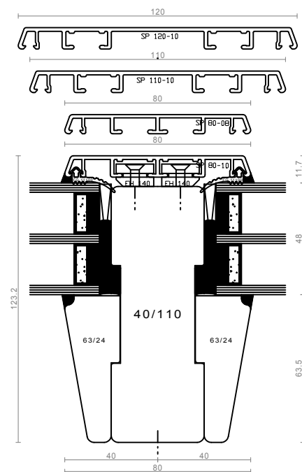
steklodeljivi križ / fiksno - horizontalni / vertikalni
