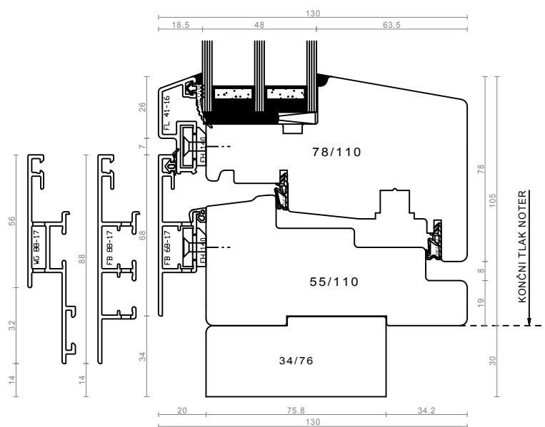
spodnji prečnik - okno in balkonska vrata
