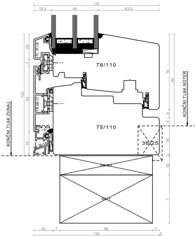
slepi podboj - spodnji prečnik - balkonska vrata
