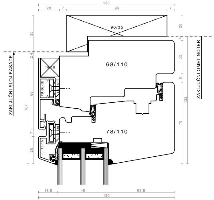
slepi podboj - pokončnik in zgornji prečnik
