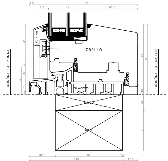
slepi podboj - spodnji prečnik - balkonska vrata / pohodni profil
