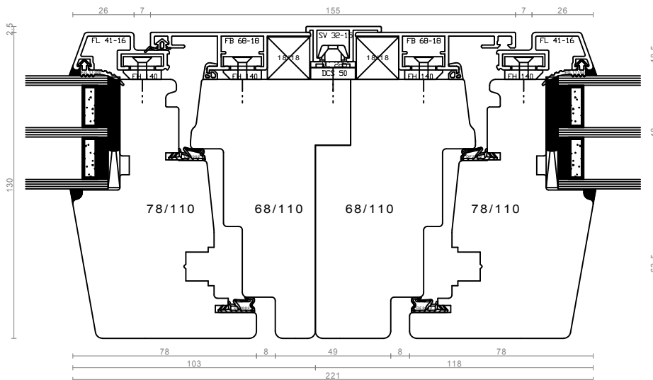
sestav po horizontali / slepi podboj - DK/DK
