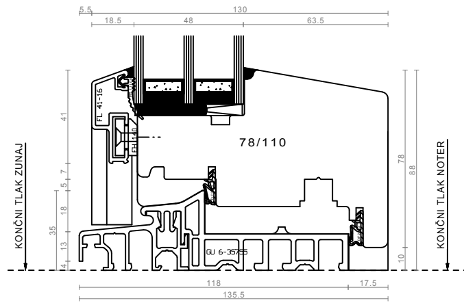
spodnji prečnik / pohodni profil - balkonska vrata
