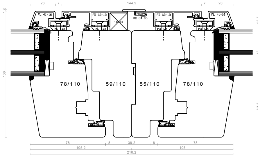
sestav po horizontali - DK/DK
