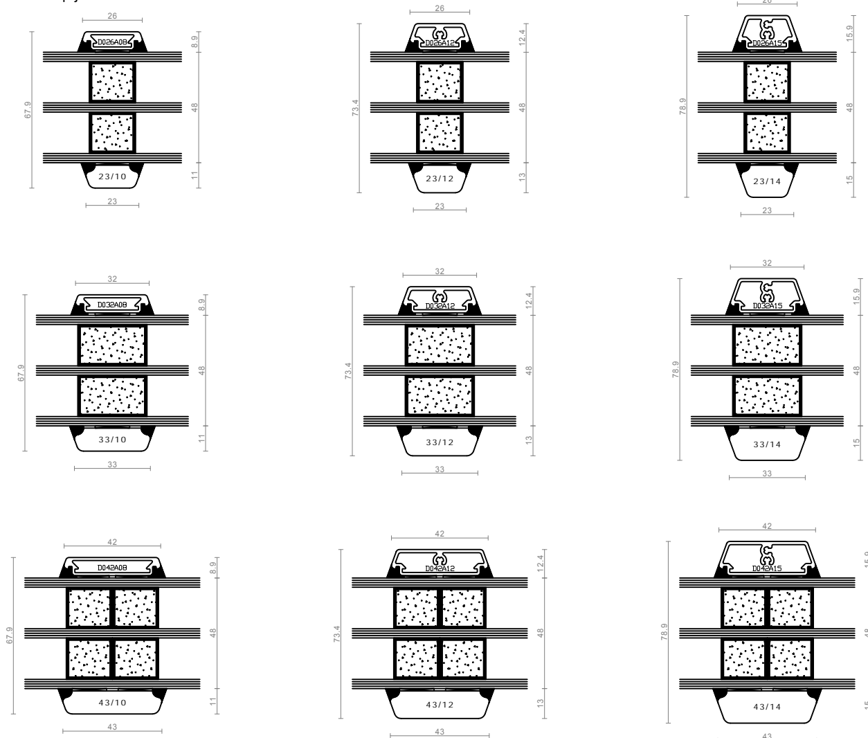
nalepljeni križi - horizontalni / vertikalni
