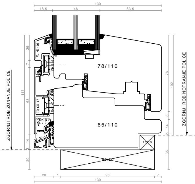
slepi podboj - spodnji prečnik - okno
