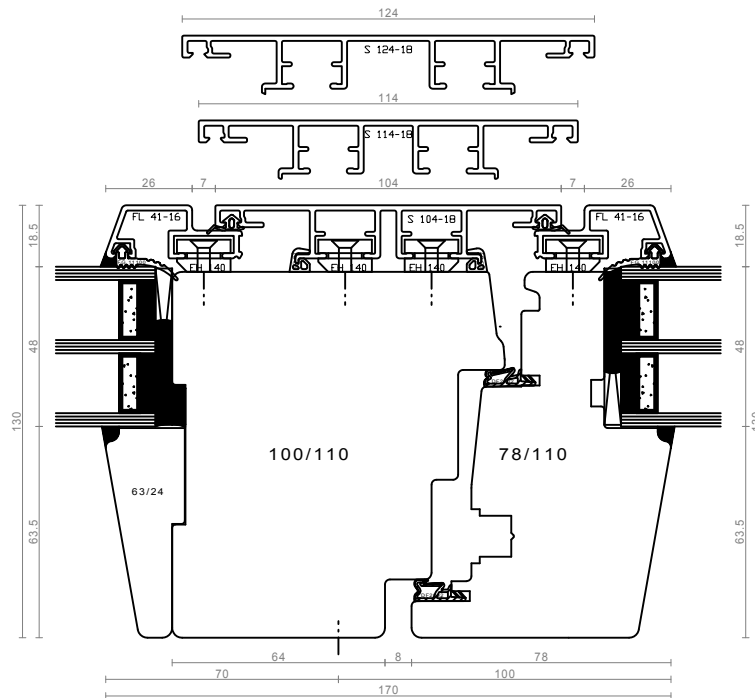
sredinski pokončnik - FIX/DK
