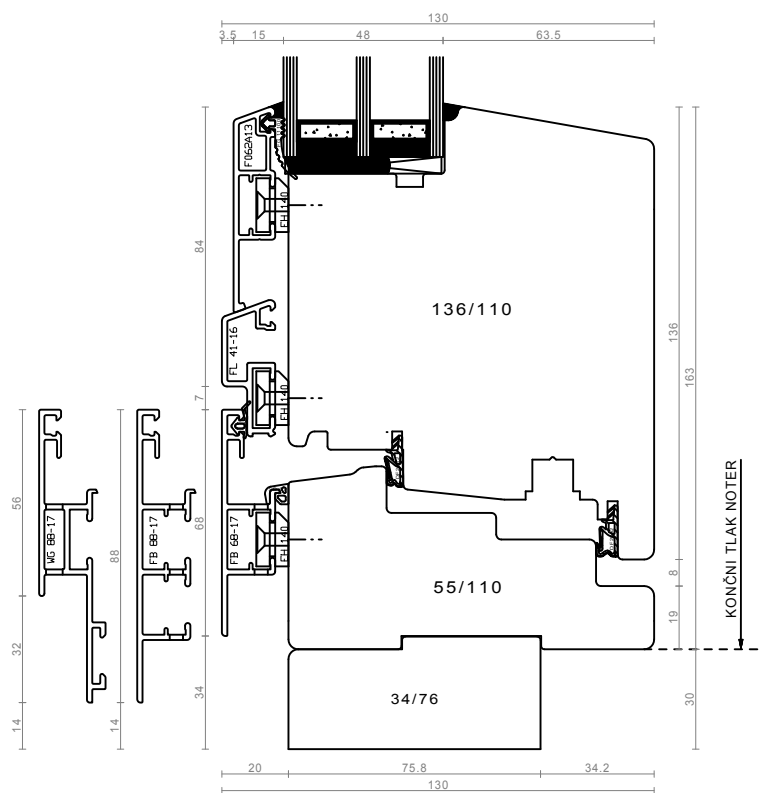
spodnji prečnik - balkonska vrata (razširano)
