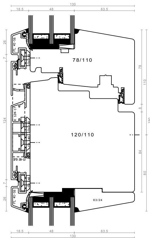
sredinski prečnik - DK/FIX
