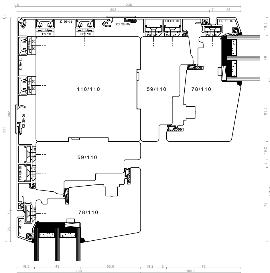
vogalni sestav - DK/DK
