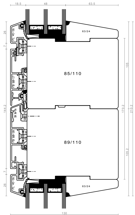
sestav po vertikali - FIX/FIX
