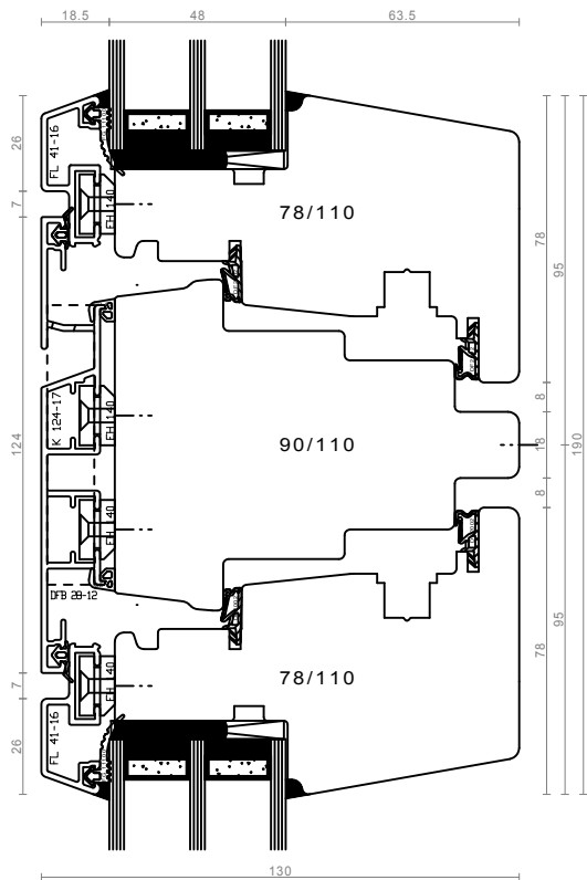
sredinski prečnik - KIP/DK
