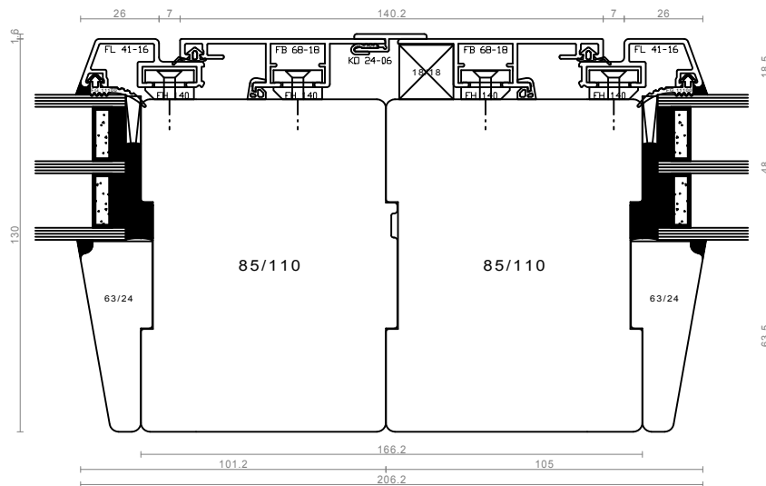
sestav po horizontali - FIX/FIX
