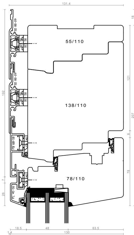
vložek v okvirju - pokončnik in zgornji prečnik
