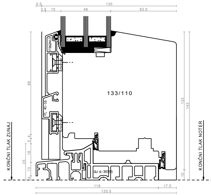
spodnji prečnik / pohodni profil - balkonska vrata (razširano)
