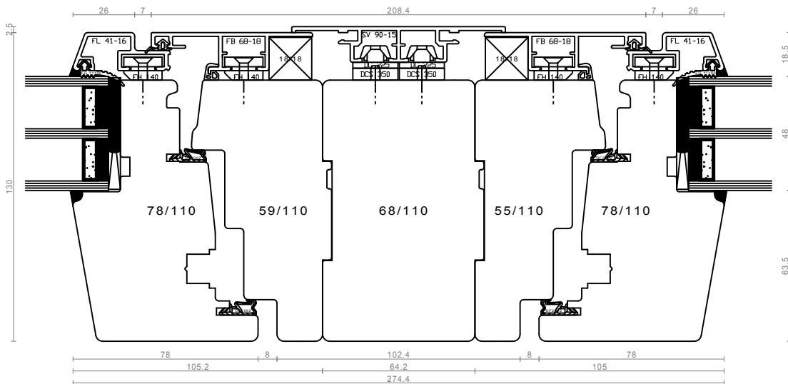
sestav po horizontali z vmesnim vložkom - DK/DK
