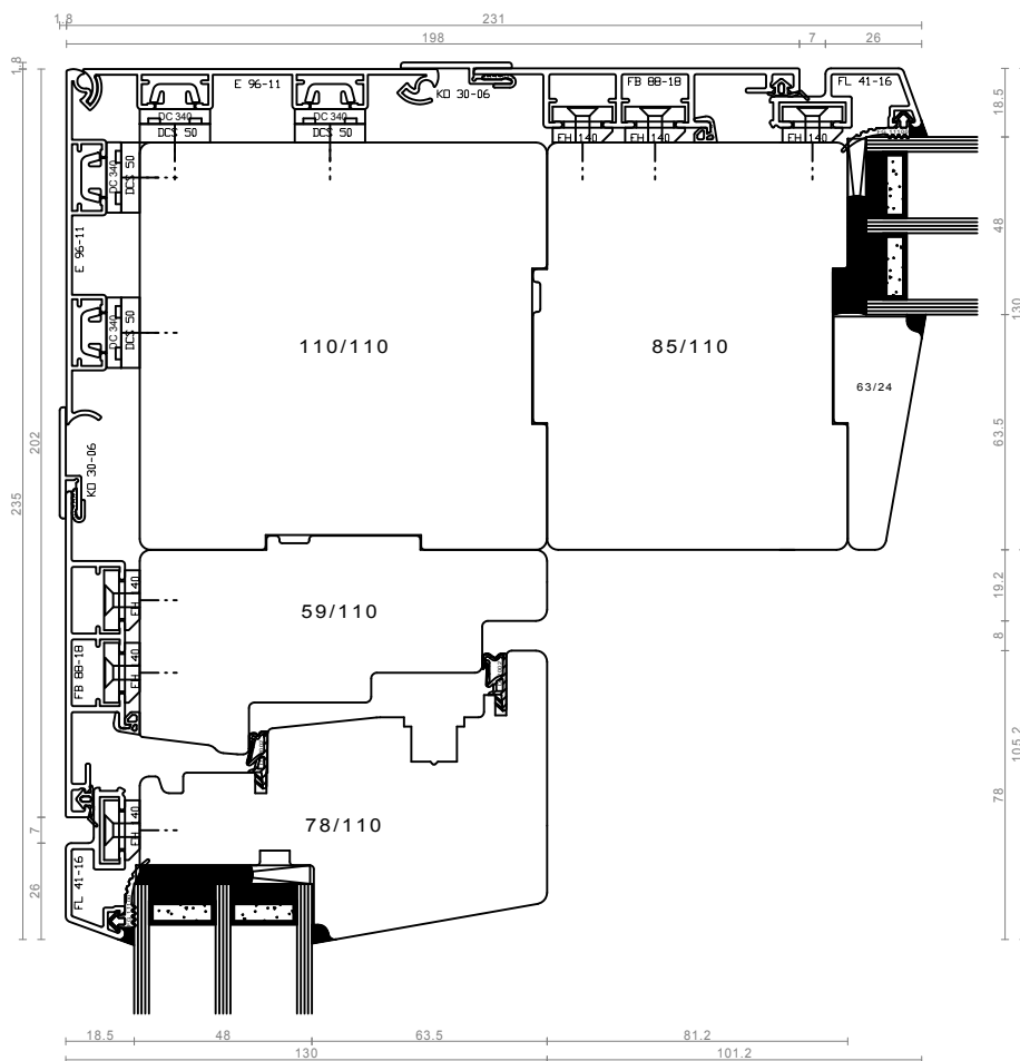
vogalni sestav - DK/FIX
