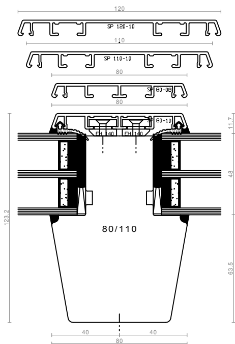
steklodeljivi križ / krilo - horizontalni / vertikalni
