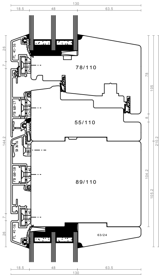
sestav po vertikali - DK/FIX
