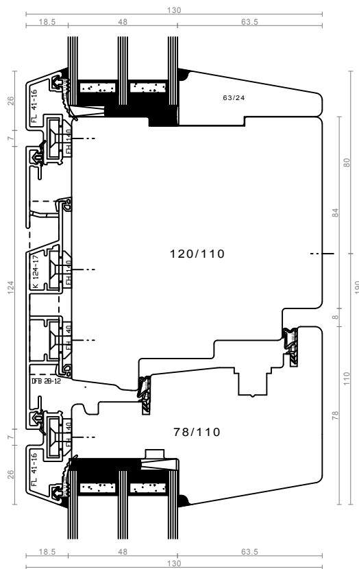
sredinski prečnik - FIX/DK
