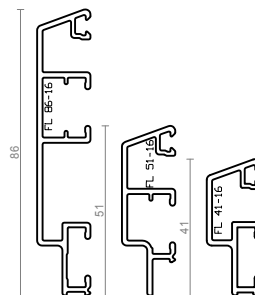
Alu obloga za krilo
