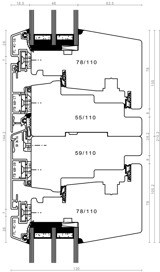
sestav po vertikali - DK/DK
