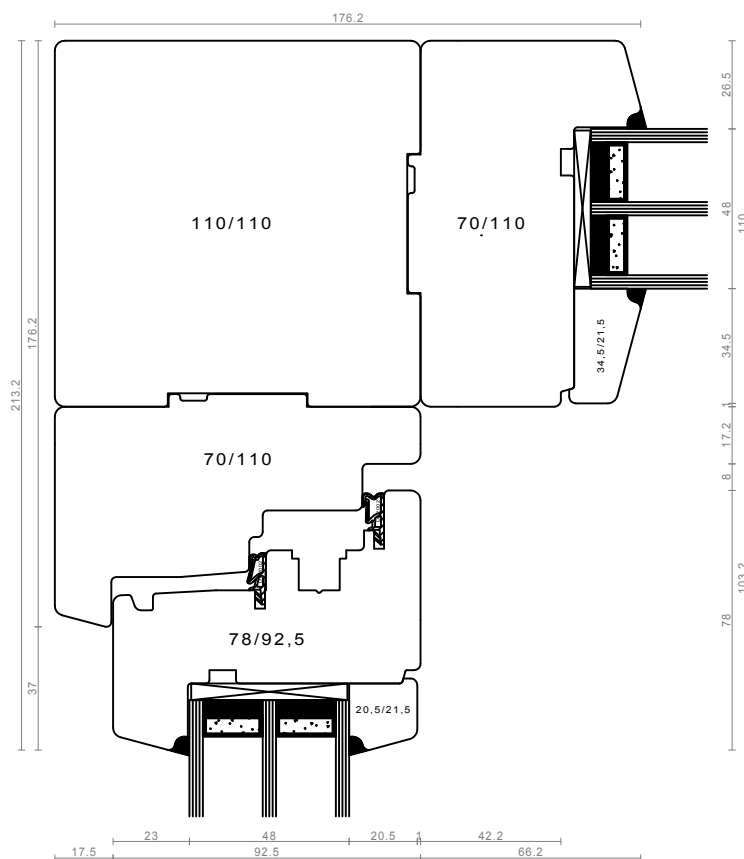
vogalni sestav - DK/FIX
