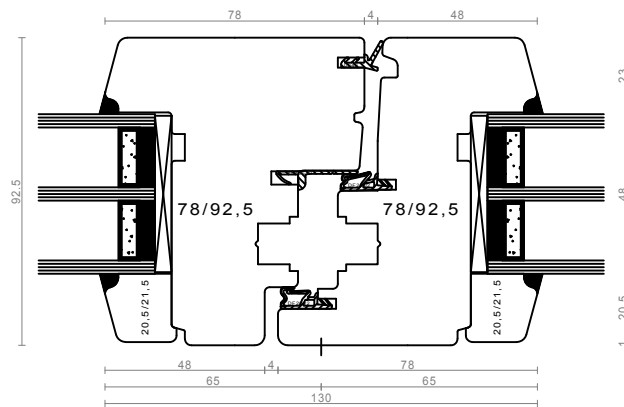
dvokrilno brez pokončnika - D/DK
