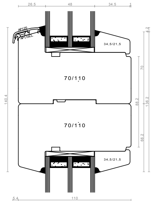
sestav po vertikali - FIX/FIX
