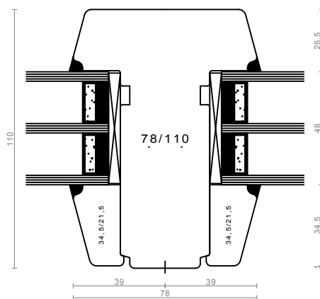
steklodeljivi križ / fiksno - horizontalni / vertikalni
