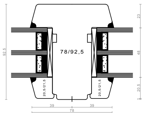
steklodeljivi križ / krilo - horizontalni / vertikalni
