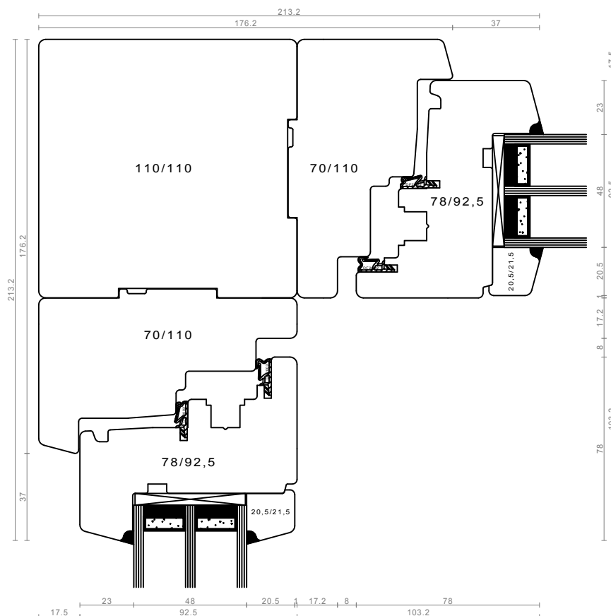
vogalni sestav - DK/DK
