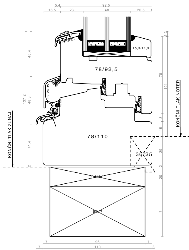
slepi podboj - spodnji prečnik - balkonska vrata
