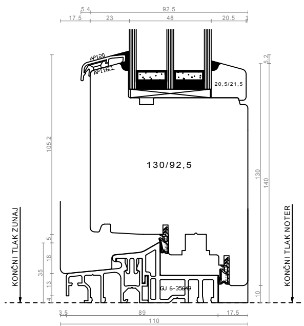
spodnji prečnik / pohodni profil - balkonska vrata (razširano)
