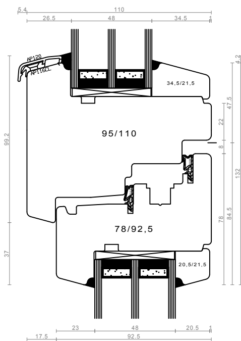
sredinski prečnik - FIX/DK
