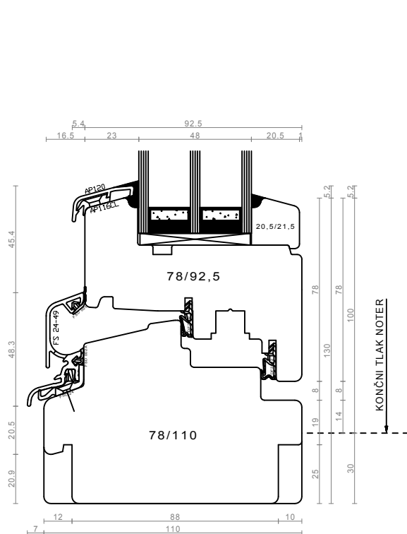
spodnji prečnik - okno in balkonska vrata
