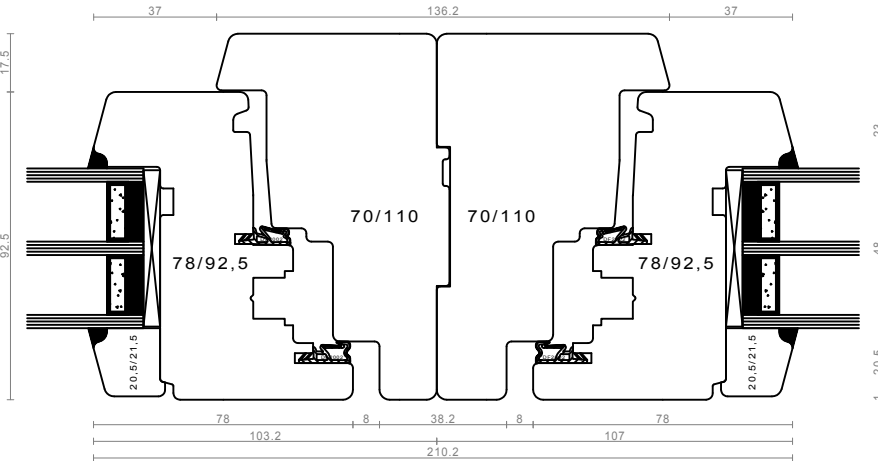
sestav po horizontali - DK/DK
