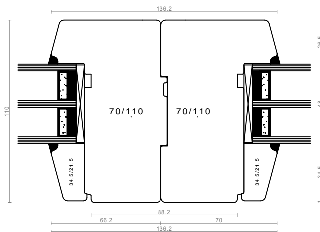
sestav po horizontali - FIX/FIX
