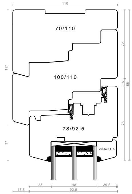
vložek v okvirju - pokončnik in zgornji prečnik
