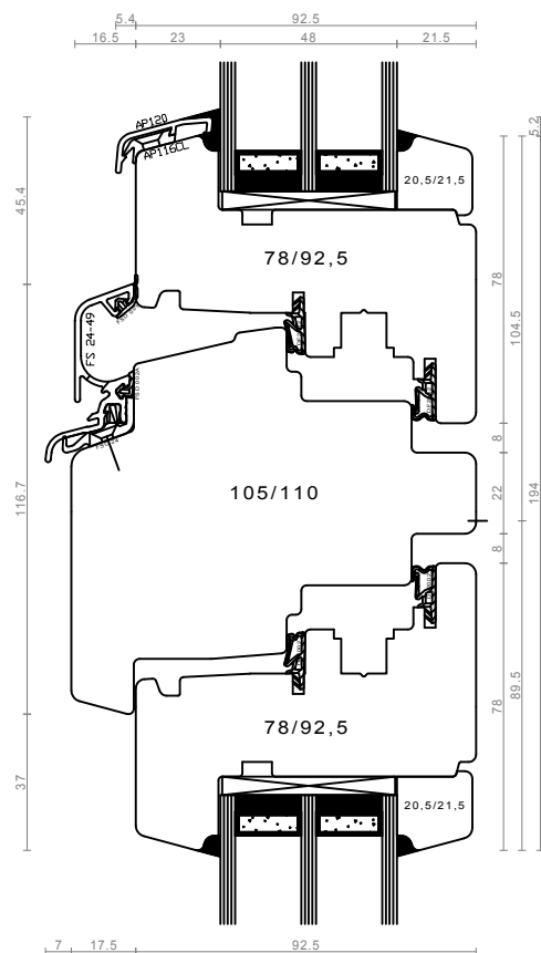
sredinski prečnik - KIP/DK
