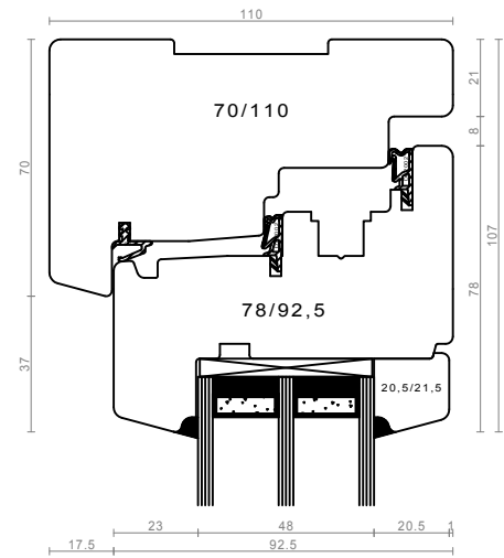
pokončnik in zgornji prečnik - tretje tesnilo
