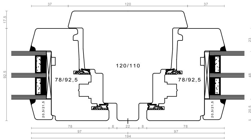
dvokrilno s pokončnikom - DK/DK
