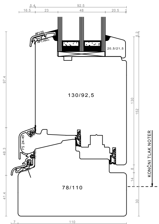
spodnji prečnik - balkonska vrata (razširano)
