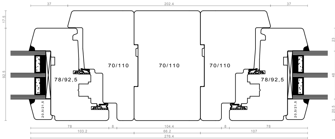
sestav po horizontali z vmesnim vložkom - DK/DK
