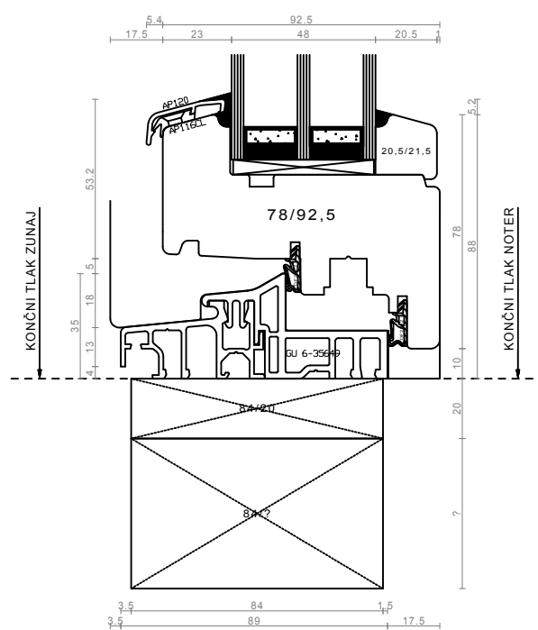
slepi podboj - spodnji prečnik - balkonska vrata / pohodni profil
