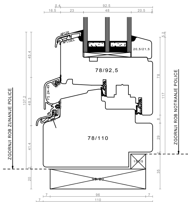
slepi podboj - spodnji prečnik - okno
