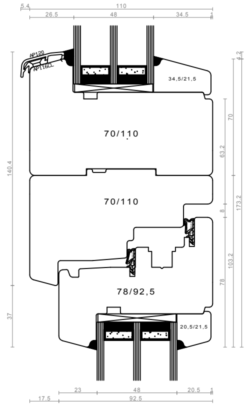
sestav po vertikali - FIX/DK
