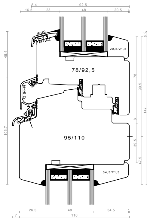
sredinski prečnik - DK/FIX
