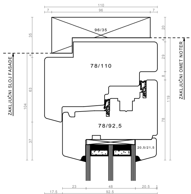
slepi podboj - pokončnik in zgornji prečnik
