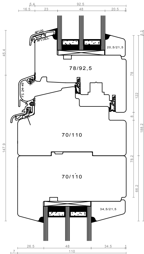
sestav po vertikali - DK/FIX
