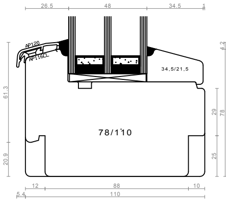
spodnji prečnik - fiksno okno
