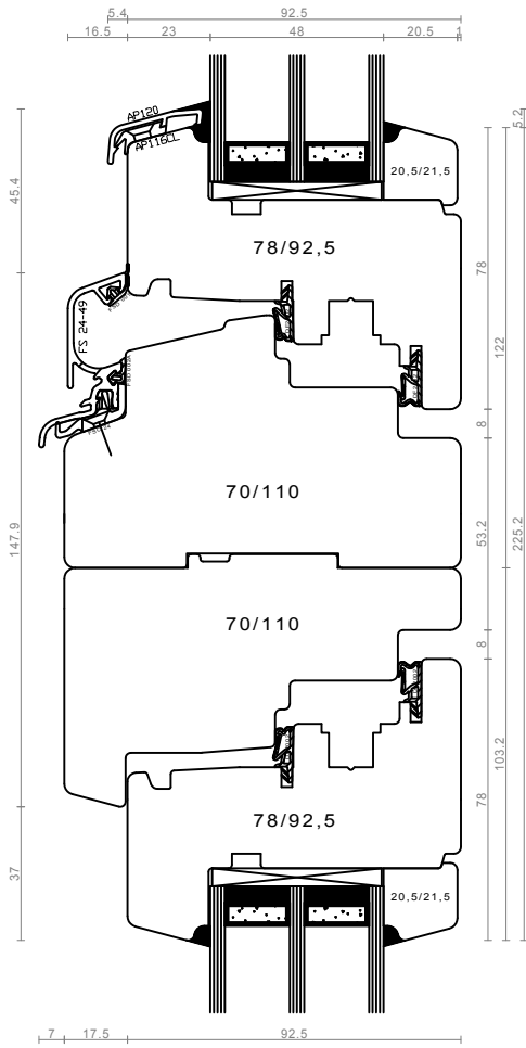
sestav po vertikali - DK/DK
