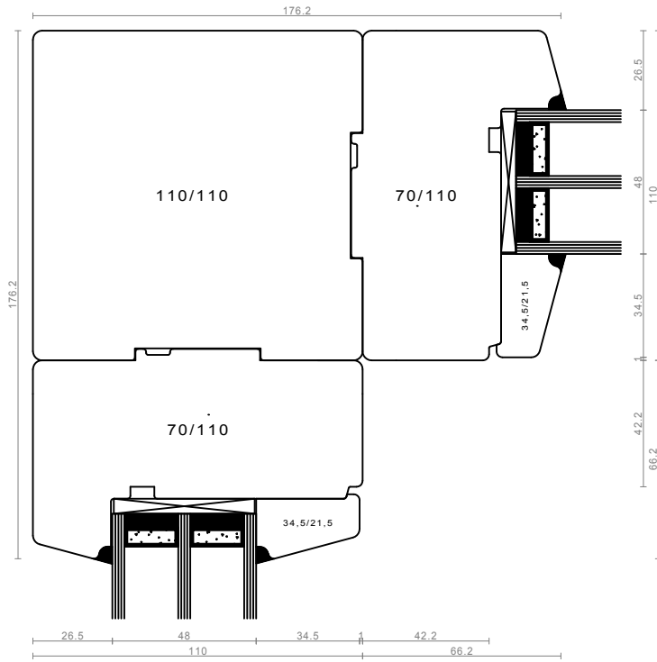
voglani sestav - FIX/FIX
