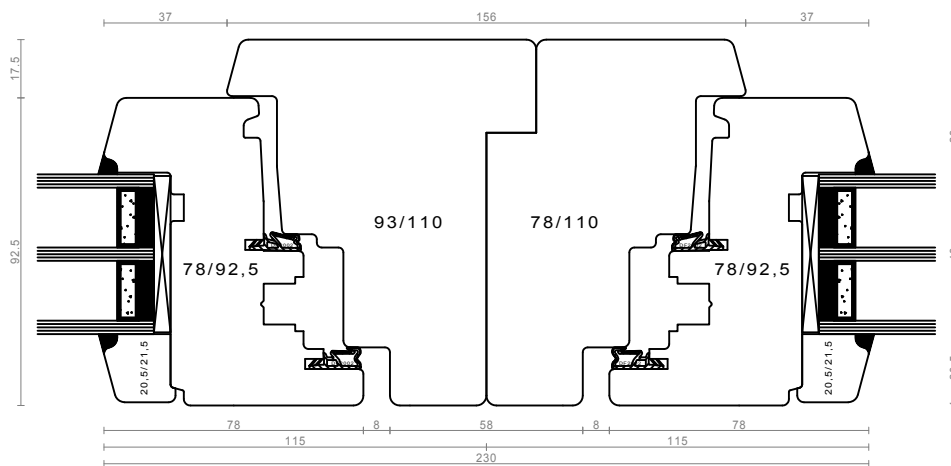
sestav po horizontali / slepi podboj - DK/DK
