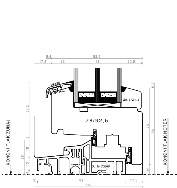
spodnji prečnik / pohodni profil - balkonska vrata
