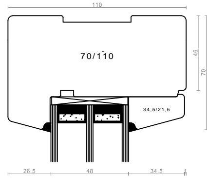
pokončnik in zgornji prečnik - fiksno okno
