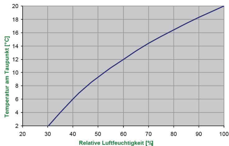
Abb. 63: Taupunkt in Abhängigkeit von der relativen Feuchtigkeit (die Ausgangstemperatur der feuchten Luft beträgt 20°C)
