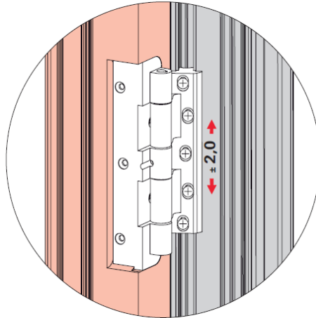
Abb. 47: Einstellung des mittleren Scharniers
