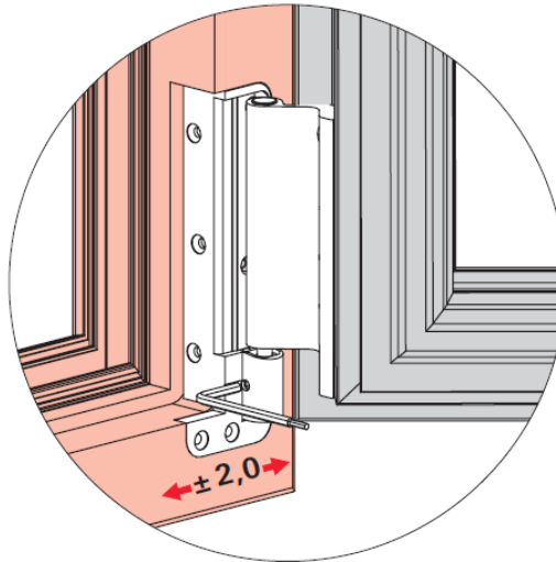
Abb. 45: Einstellung am unteren Scharnier am Rahmen
