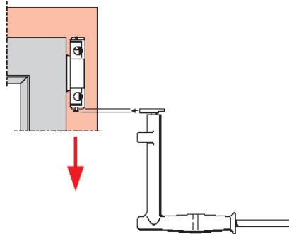
Abb. 33: Herausziehen des Bolzens
