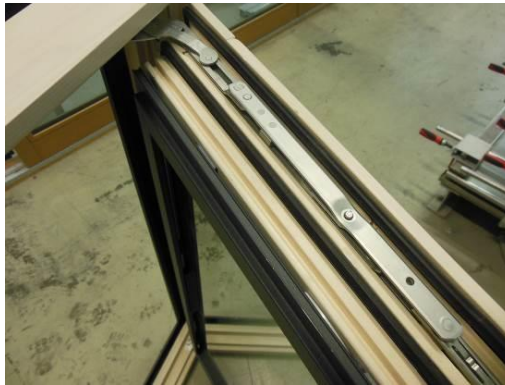
Abb. 41: Geschlossene Schere
