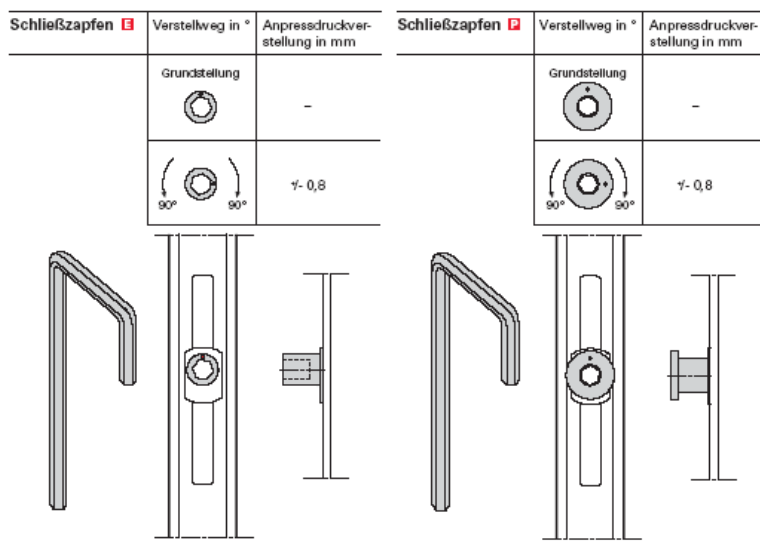
Abb. 30: Regulierung der Anpassung des Flügels auf dem Rahmen oder an das zweiflügelige Fenster
