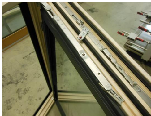
Abb. 42: Geöffnete Schere
