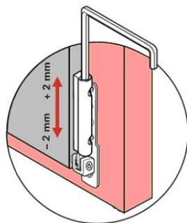
Abb. 24: Höhenverstellung der Fenster (untere Türangel)
