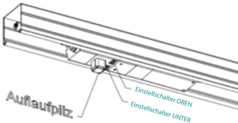
Abb. 54: Darstellung der verschiedenen Jalousien-Positionen
