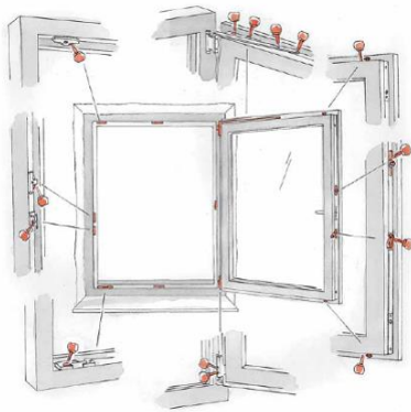
Abb. 58: Jährliches Einölen der Beschläge
