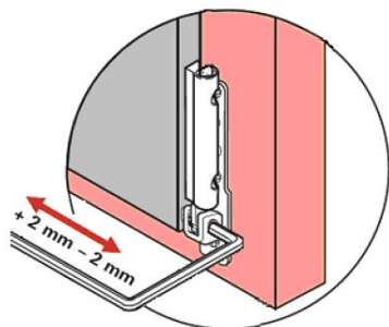
Abb. 26: Horizontale Verstellung des Fensters (untere Türangel)
