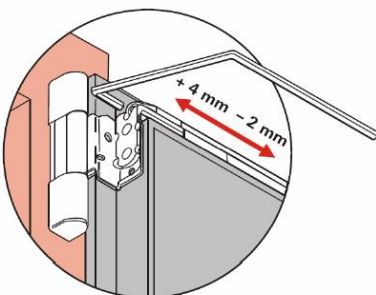
Abb. 27: Horizontale Verstellung des Fensters (obere Türangel)
