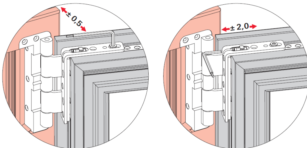
Abb. 44: Einstellung am oberen Scharnier am Rahmen in der Flügelnut
