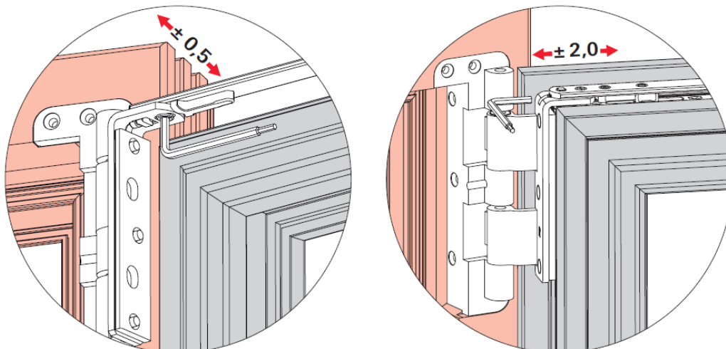
Abb. 43: Einstellung am oberen Scharnier am Rahmen
