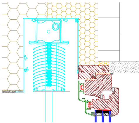
Außenjalousien
