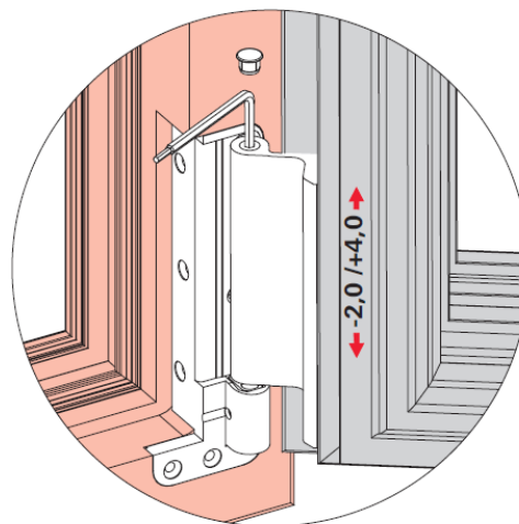
Abb. 46: Einstellung am unteren Scharnier in der Flügelnut
