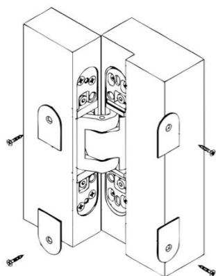
Abb. 53: Einstellung der verdeckt liegenden Scharniere der Eingangstür
