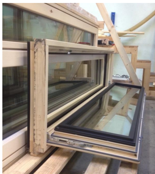
Abb. 51: Endposition – der Fensterflügel muss gestützt werden
