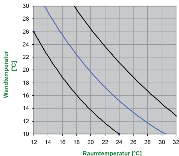
Abb. 64: Graph mit den günstigen Temperatur bereichen
